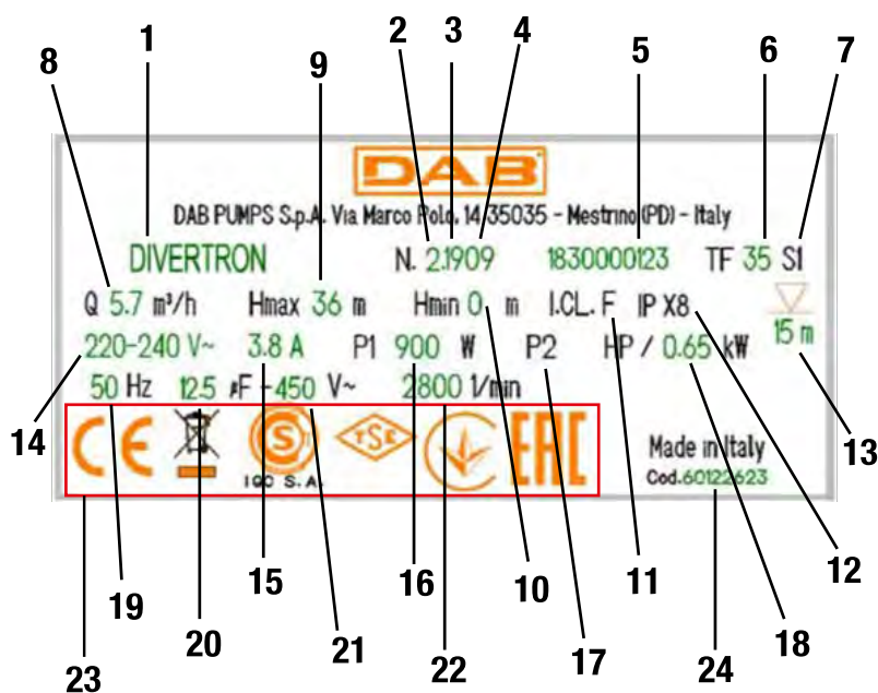
Rys. 4 Tabliczka znamionowa
