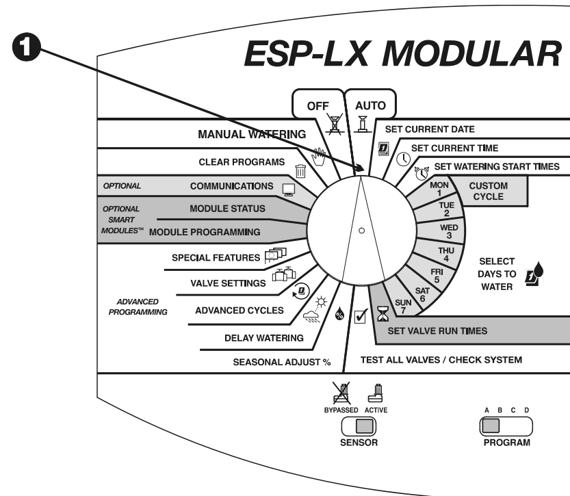
Programmeur ESP-LX modulaire
