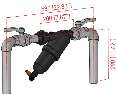
Schéma d'installation type
