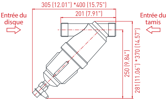
Schémas avec dimensions
