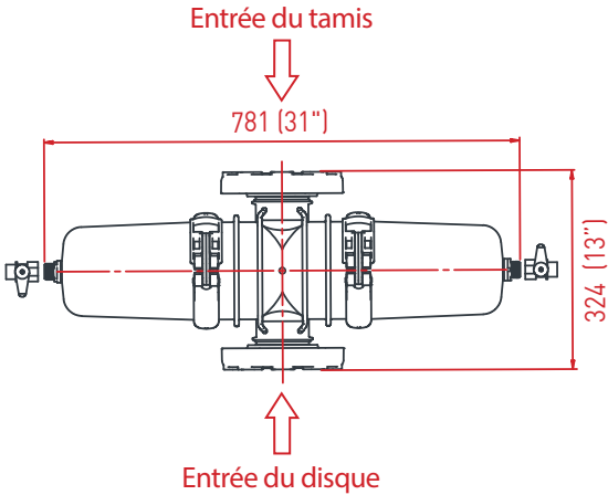
Schémas avec dimensions
