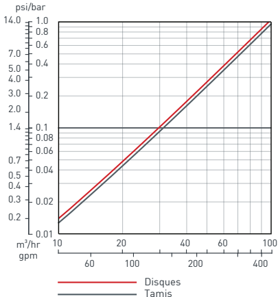
Graphique de perte de charge (avec de l'eau claire)
