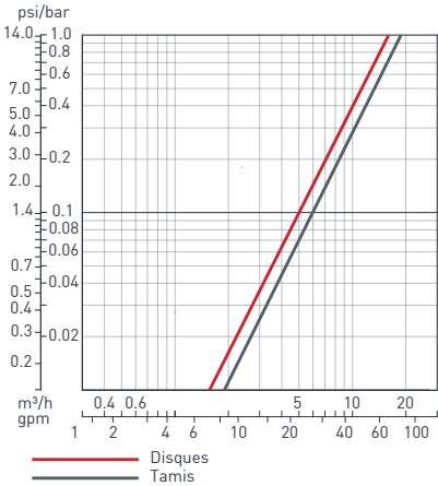
Graphique de perte de charge (avec de l'eau claire)
