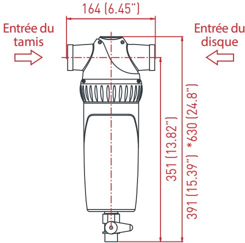
Schémas avec dimensions
