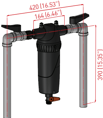
Schéma d'installation type
