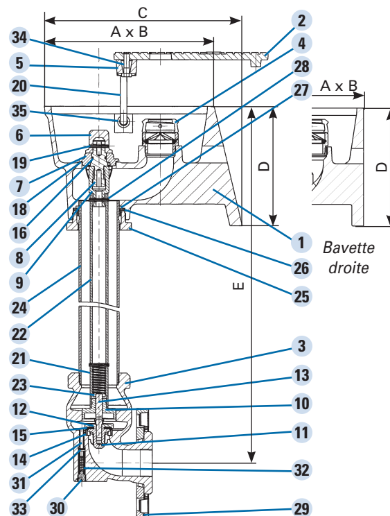
Version incongelable - bavette inclinée
