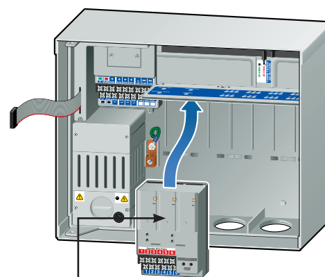
Module de sortie ADM99
