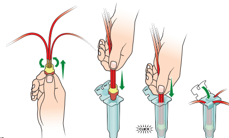
Connecteurs étanches à l'eau
