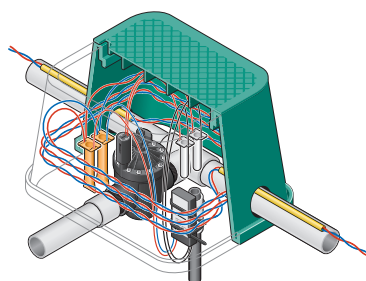
Décodeur dans regard d'électrovanne
