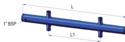
COLLETTORE DOPPIO 2 USCITA DOUBLE MANIFOLD 2 OUTLET COLLECTEUR DOUBLE 2 SORTIE COLECTORES DOBLES 2 SALIDA
